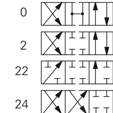
DG4V-3(S)-*ALV
