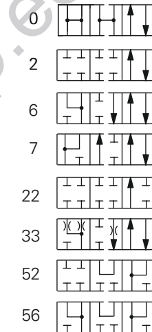
DG4V-3(S)-*BLV
