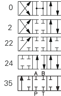
DG4V-3(S)-*BV
