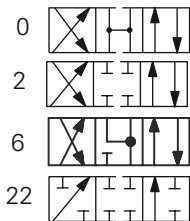
DG4V-3(S)-*NV
