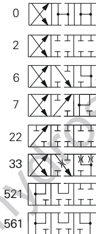
DG4V-3(S)-*BV
